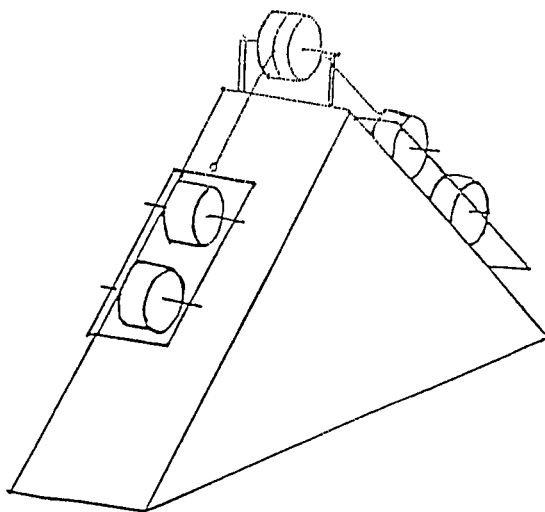
圖二 斜坡物體下滑實驗器材裝置
