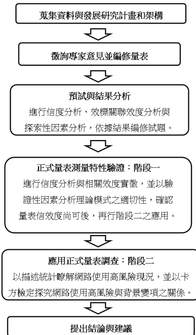
圖 1 研究流程圖
